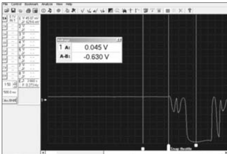
Осциллограмма выходного напряжения лямбда-зонда BOSCH (на основе оксида циркония).
