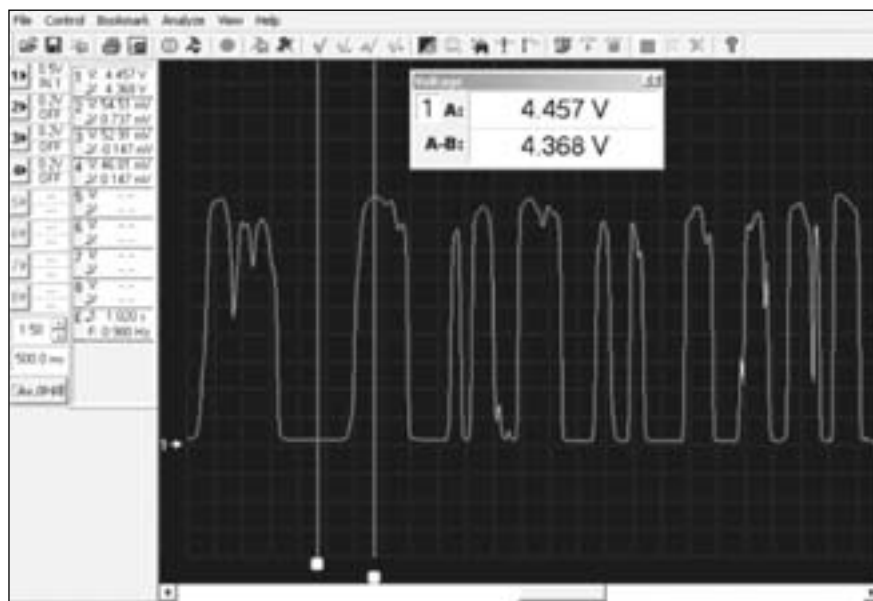
Осциллограмма выходного напряжения лямбда-зонда SIEMENS (на основе оксида титана).
