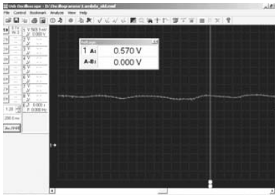
Осциллограмма выходного напряжения лямбда-зонда BOSCH (на основе оксида циркония). A: - значение напряжения в момент времени указанный маркером. В данном случае соответствует среднему значению напряжения выходного сигнала лямбда-зонда, и равно ~550mV.
