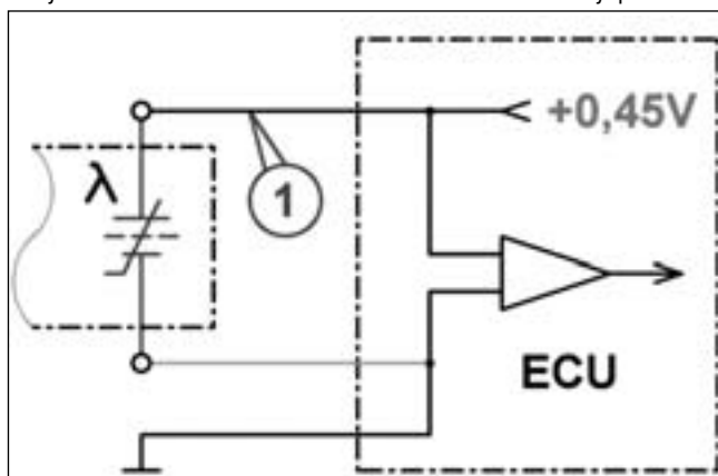
Схема подключения лямбда-зонда BOSCH (на основе оксида циркония). 1 - точка подключения щупа осциллографа для получения осциллограммы выходного сигнала датчика.
