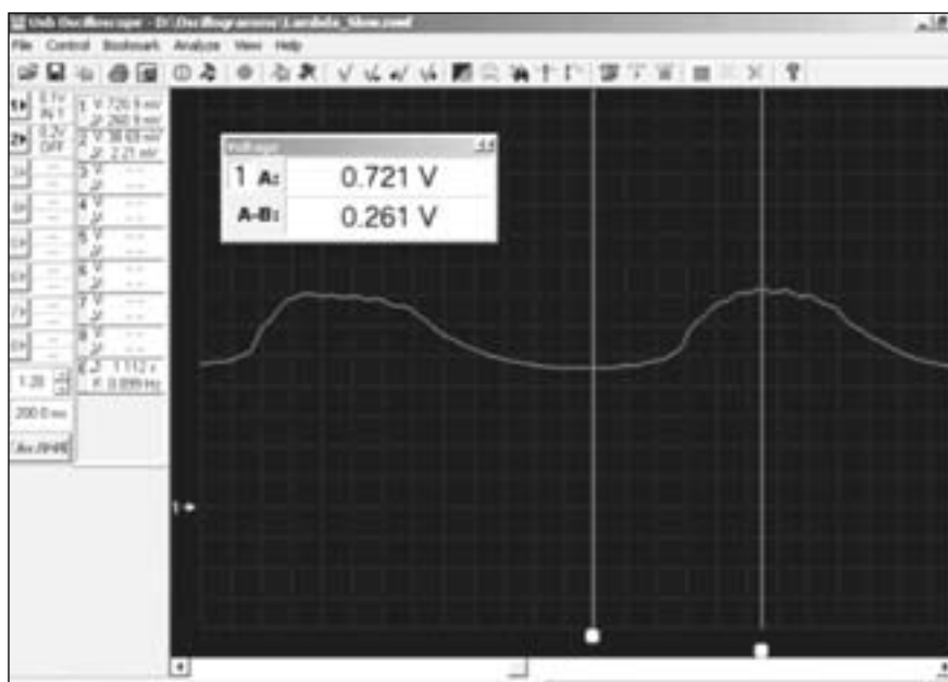
Осциллограмма выходного напряжения лямбда-зонда BOSCH (на основе оксида циркония). A: - значение напряжения в момент времени указанный маркером. В данном случае соответствует максимальному напряжению выходного сигнала лямбда-зонда и равно ~720mV; A-B: - значение разности напряжений между двумя указанными маркерами моментами времени. В данном случае соответствует размаху выходного напряжения сигнала зонда и равно ~260mV.
